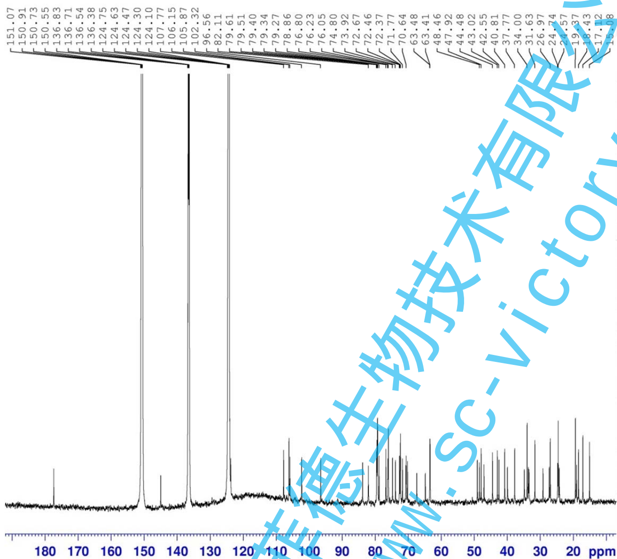
13 C-NMR 图
